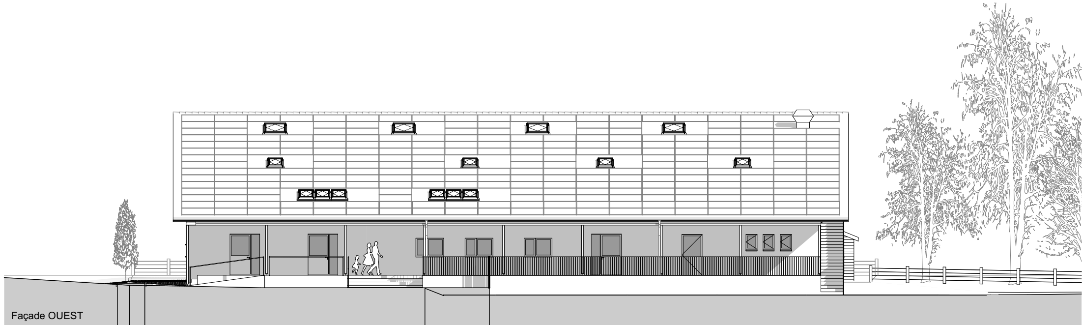
Façade SUD
